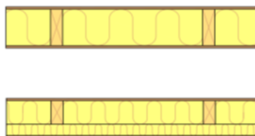
Kuva 4. Esimerkkejä ulkoseinärakenteen korjaustasoista (Puuinfo Oy, Puurakenteen_U-arvo_versio_1-03)
