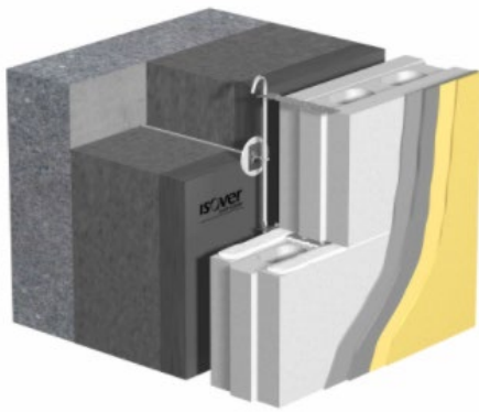
Kuva 9. Kahi Facade -julkisivu
