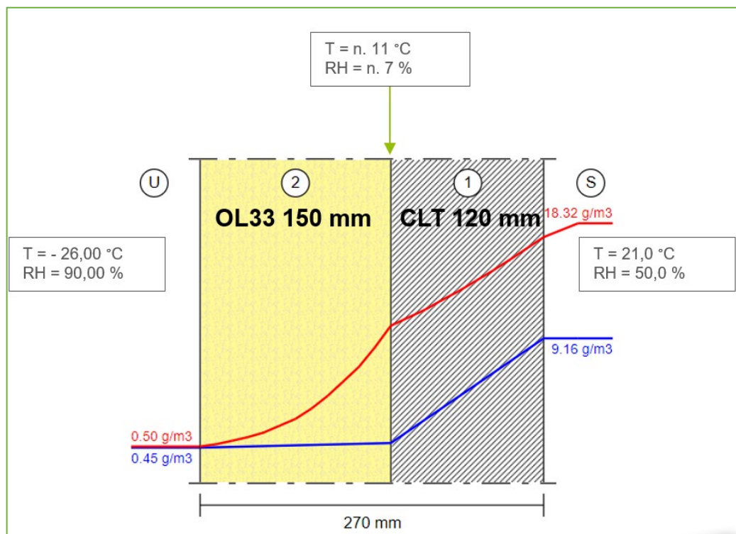
Kuva 11. Ulkopuolelta lämmöneristetty CLT-rakenne ilman höyrynsulkukalvoa.
