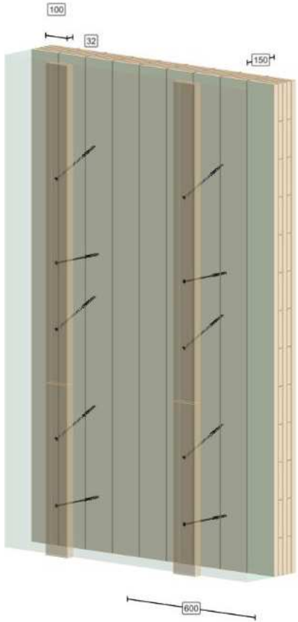
Ruuvauksen havainnollistava 3D -kuva (SPAX Design Software)
